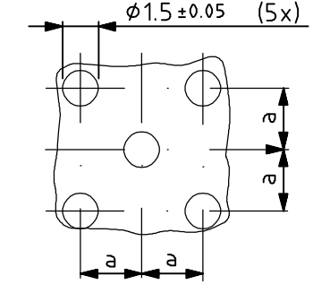
LEITERPLATTENBOHRBILD PC-BOARD LAYOUT
